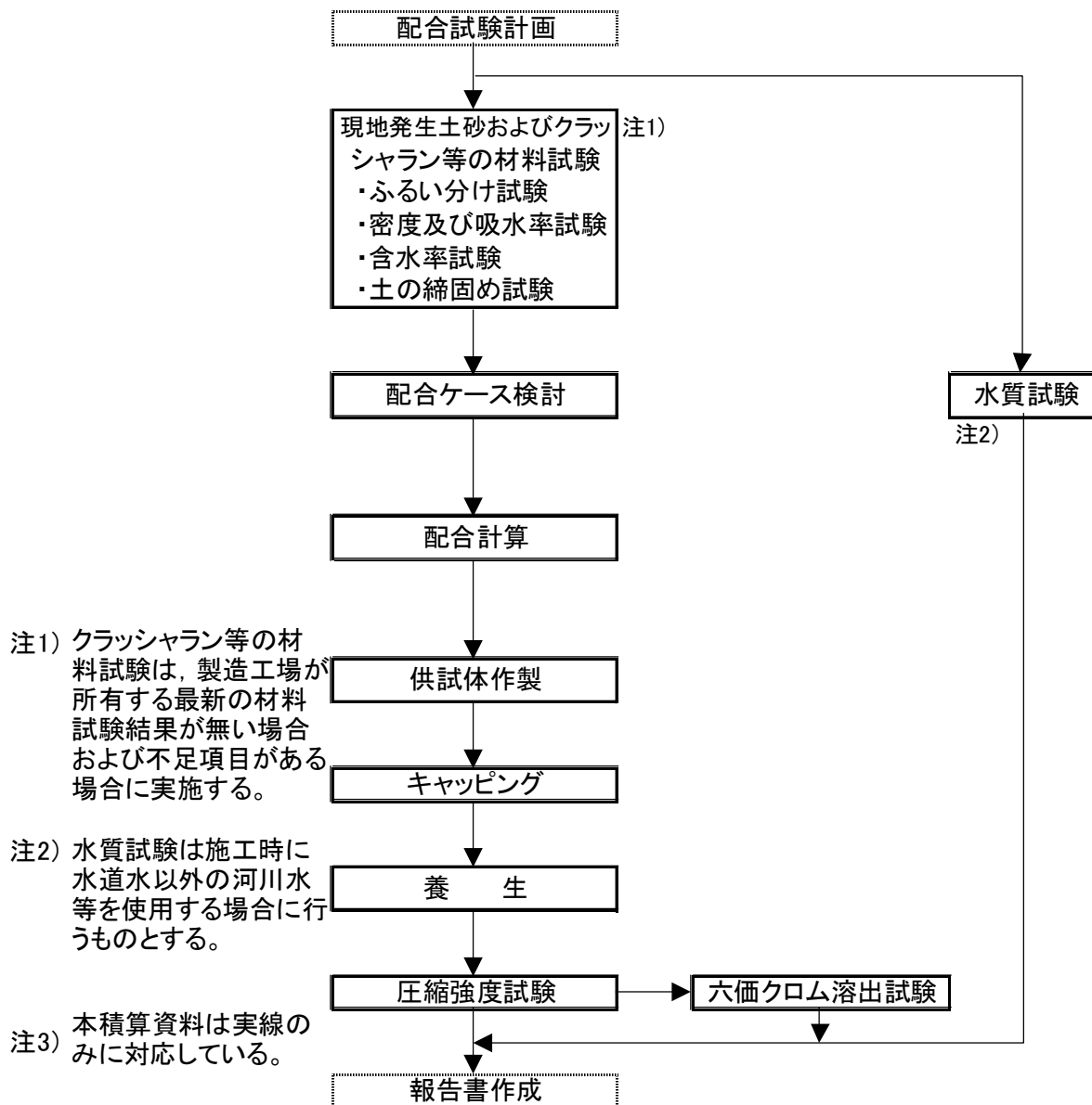
図- 2.1 作業フロー
